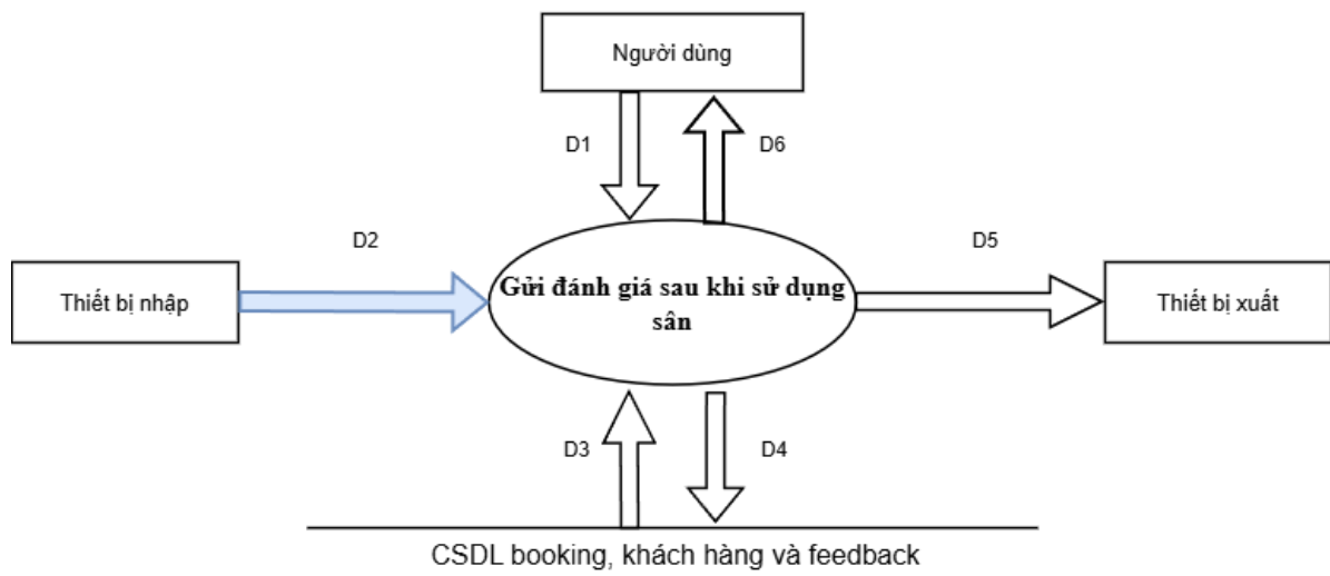
Hình DFD 2.12.1. Gửi đánh giá sau khi sử dụng sân
