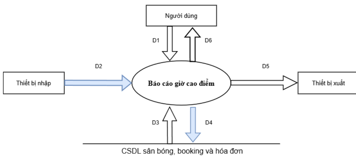
Hình DFD 2.13.3. Báo cáo giờ cao điểm
