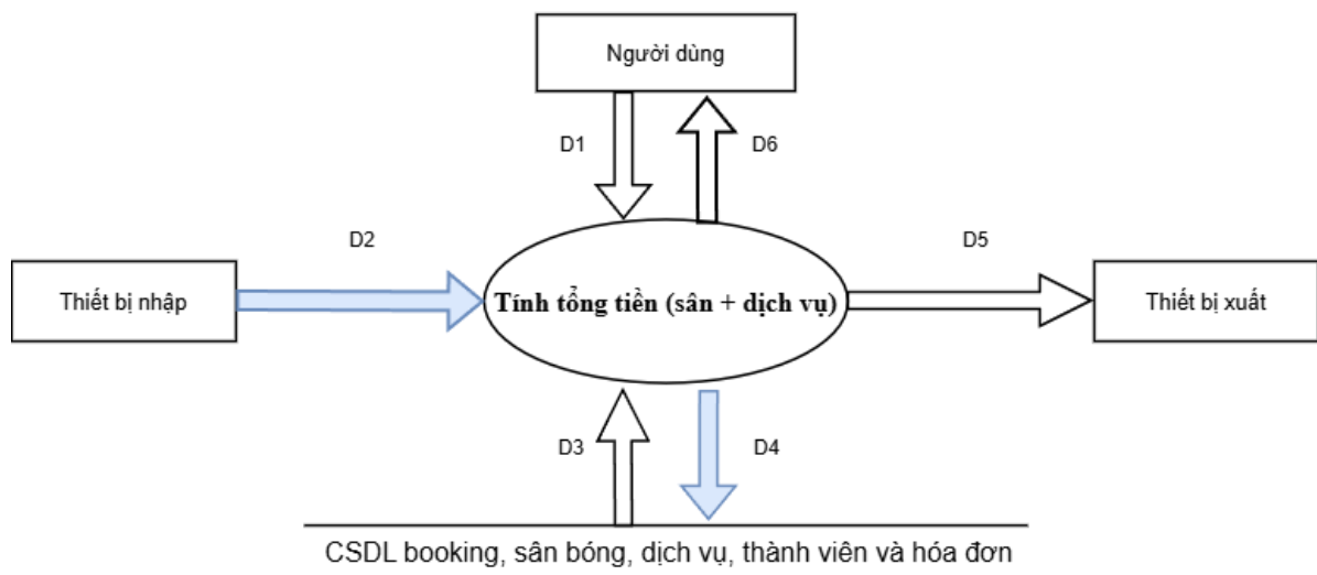
Hình DFD 2.9.1. Tính tổng tiền (sân + dịch vụ)
