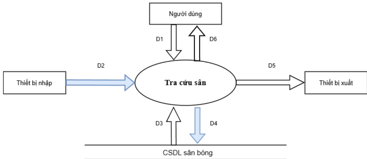
Hình DFD 2.5.2 Tra cứu sân
