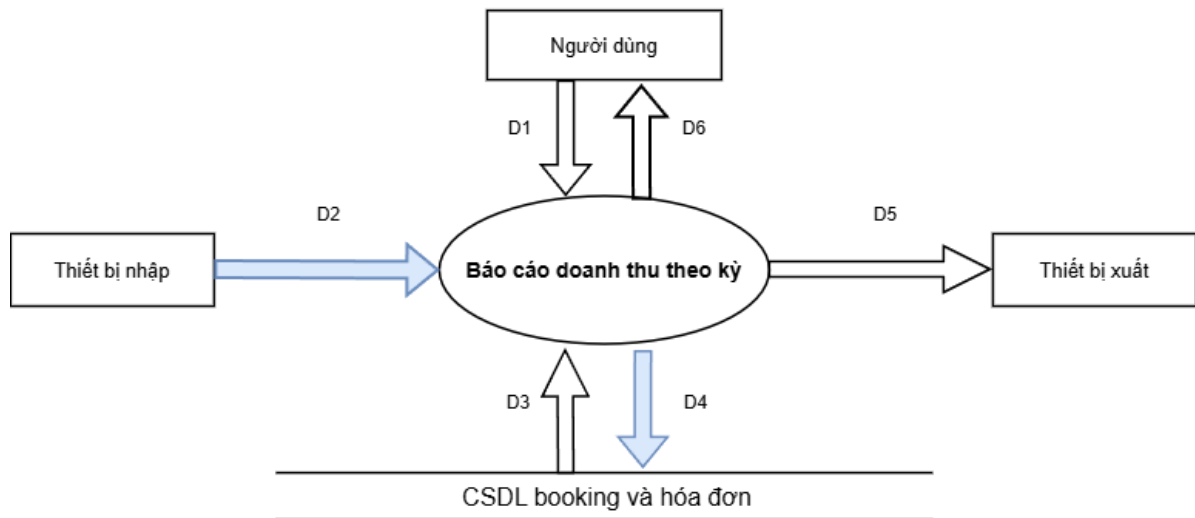
Hình DFD 2.13.1. Báo cáo doanh thu theo kỳ
