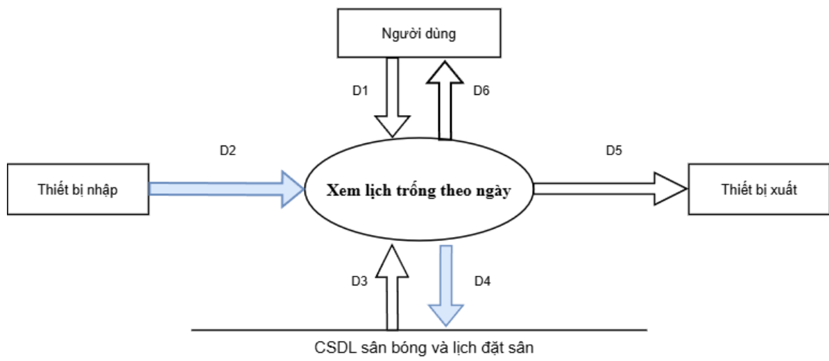
Hình DFD 2.6.1. Xem lịch trống theo ngày
