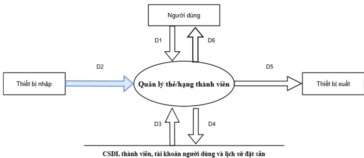
Hình DFD 2.7.1 Quản lý thẻ/hạng thành viên
