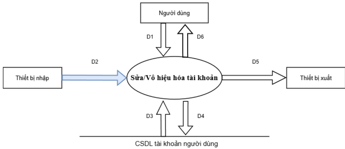
Hình DFD 2.4.3 Sửa/Vô hiệu hóa tài khoản
