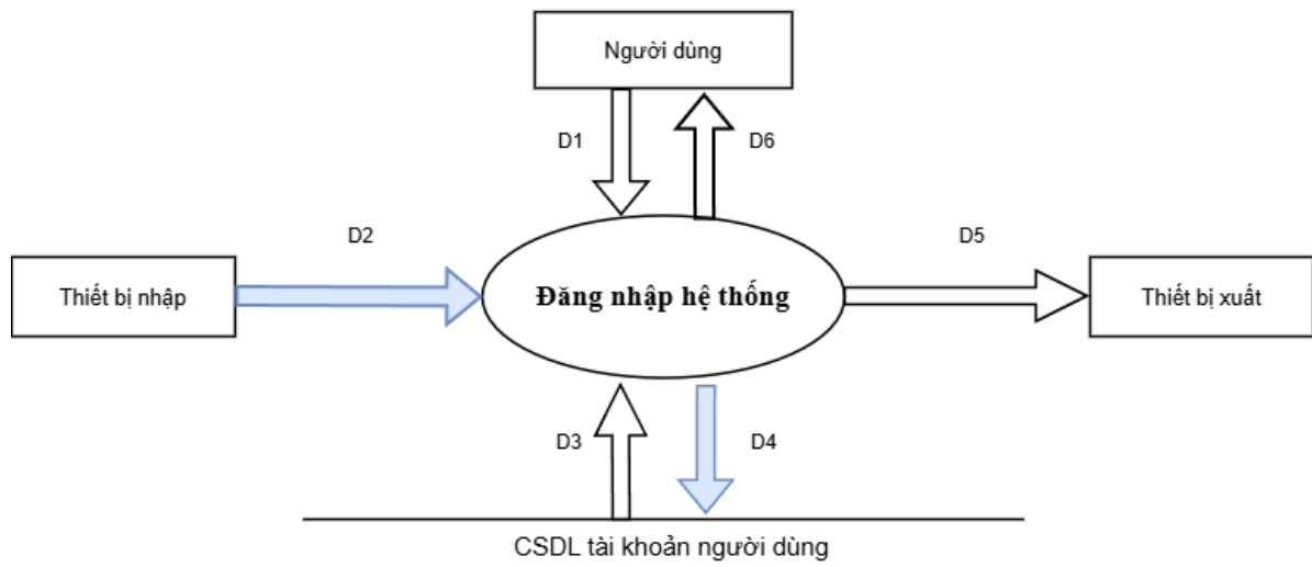
Hình DFD 2.4.1 Đăng nhập hệ thống
