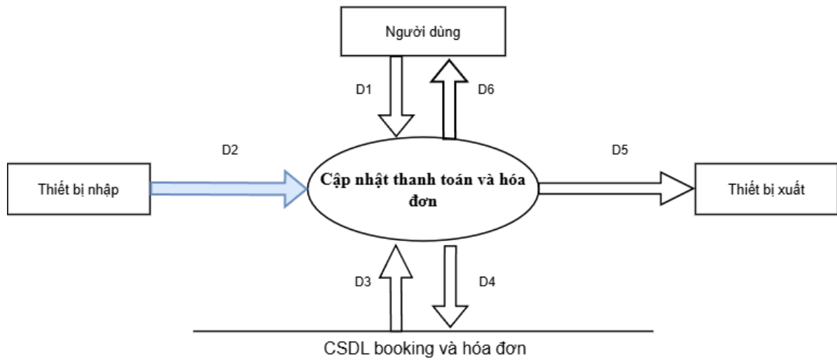
Hình DFD 2.9.2. Cập nhật thanh toán và hóa đơn
