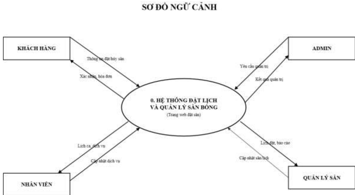
Hình 2.1. Sơ đồ ngữ cảnh hệ thống đặt lịch và quản lý sân bóng
