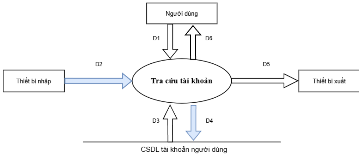
Hình DFD 2.4.4 Tra cứu tài khoản
