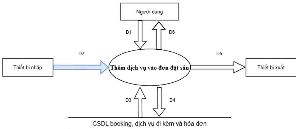
Hình DFD 2.8.2. Thêm dịch vụ vào đơn đặt sân
