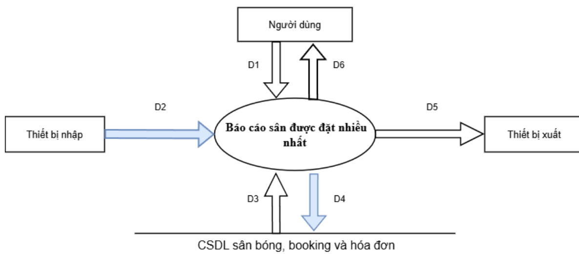
Hình DFD 2.13.2. Báo cáo sân được đặt nhiều nhất
