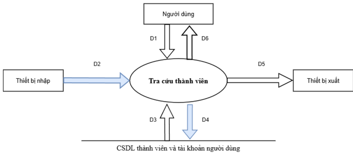
Hình DFD 2.7.2 Tra cứu thành viên
