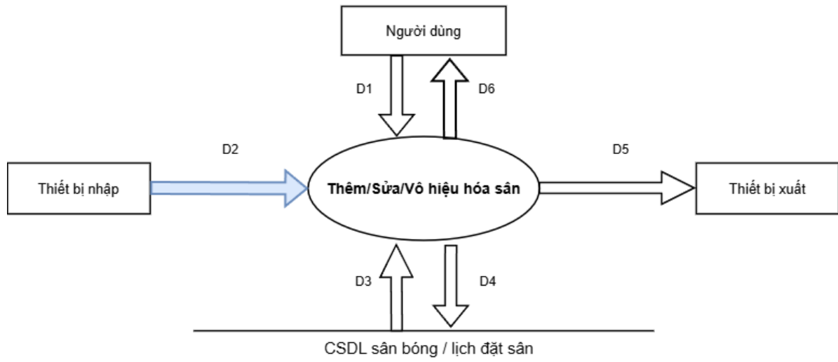
Hình DFD 2.5.1 Thêm/Sửa/Vô hiệu hóa sân
