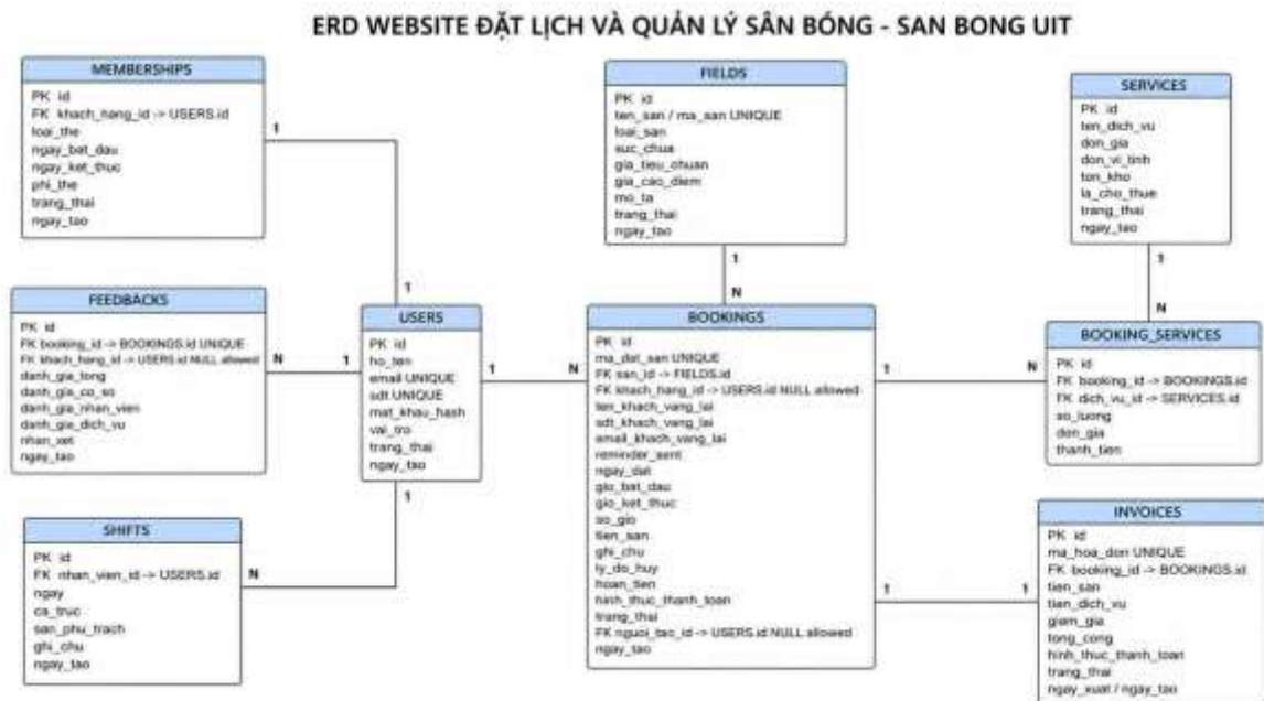
Hình 6.1. Mô hình quan hệ dữ liệu của hệ thống
