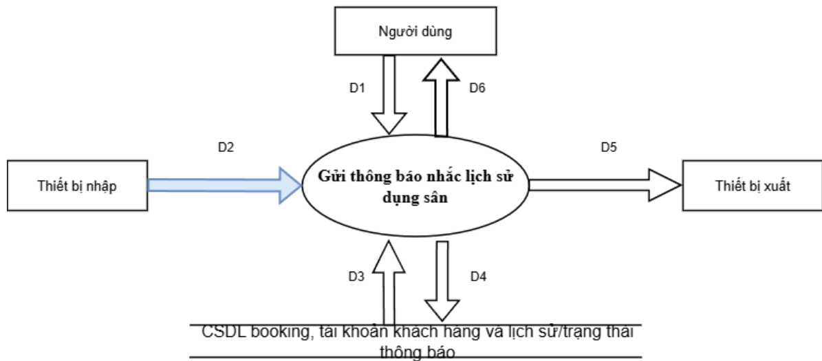
Hình DFD 2.11.1. Gửi thông báo nhắc lịch sử dụng sân
