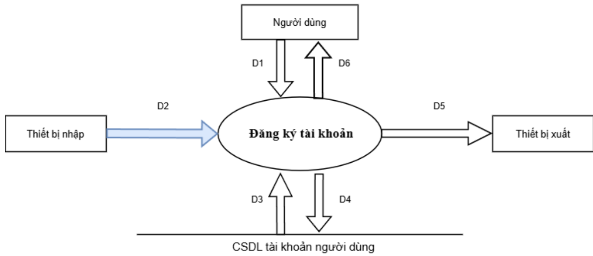
Hình DFD 2.4.2 Đăng ký tài khoản
