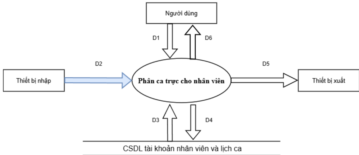
Hình DFD 2.10.1. Phân ca trực cho nhân viên
