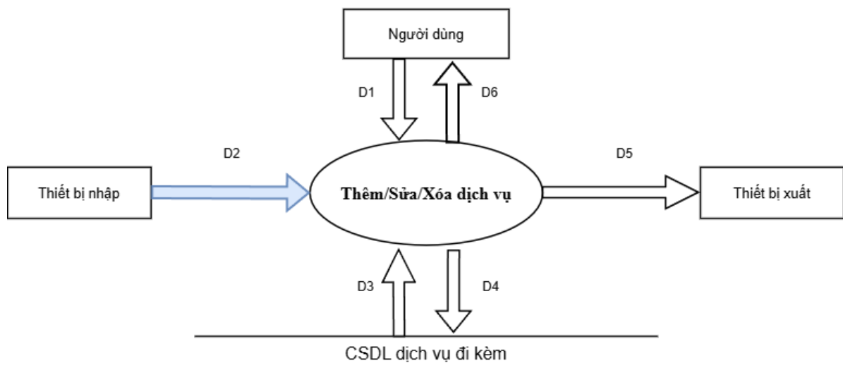
Hình DFD 2.8.1. Thêm/Sửa/Xóa dịch vụ
